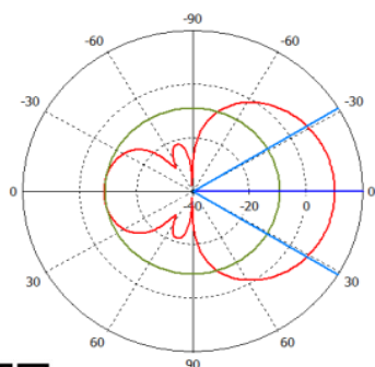
Е-плоскость (Horwin AP1800V)
