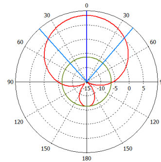
H-площина (Horwin AP800)
