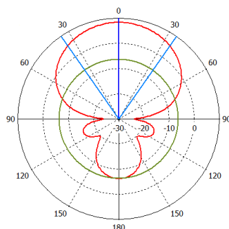
E-площина (Horwin AP800)
