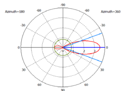
H-plane (Horwin AD 1602)
