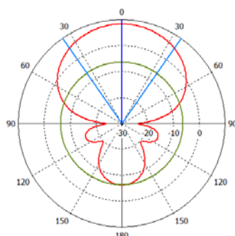
Е-плоскость (Horwin AP800)
