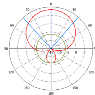
Н-плоскость (Horwin AP800)
